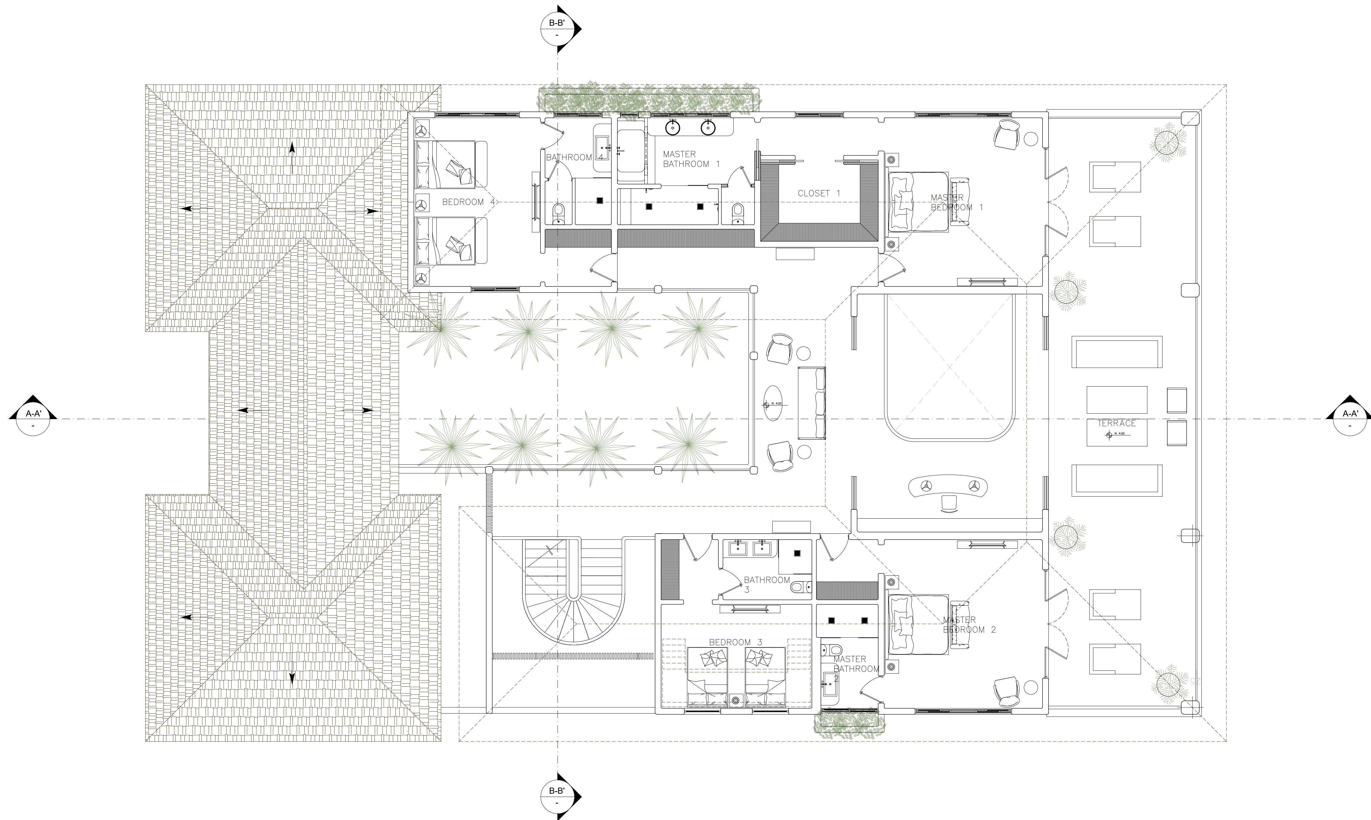
PLANTA ARQUITECTONICA SEGUNDO NIVEL ESC. 1:75
