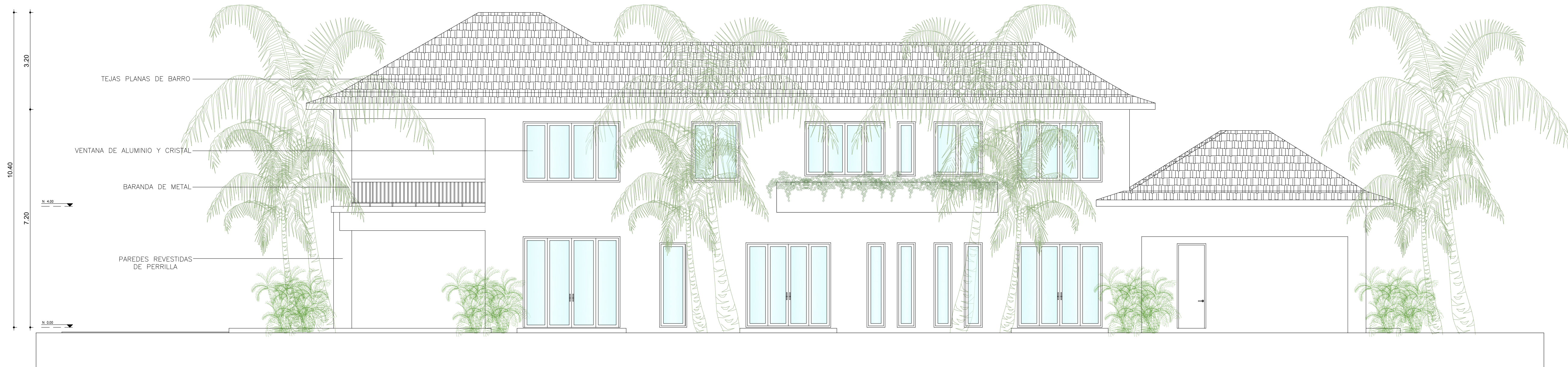
ELEVACION LATERAL IZQUIERDO
